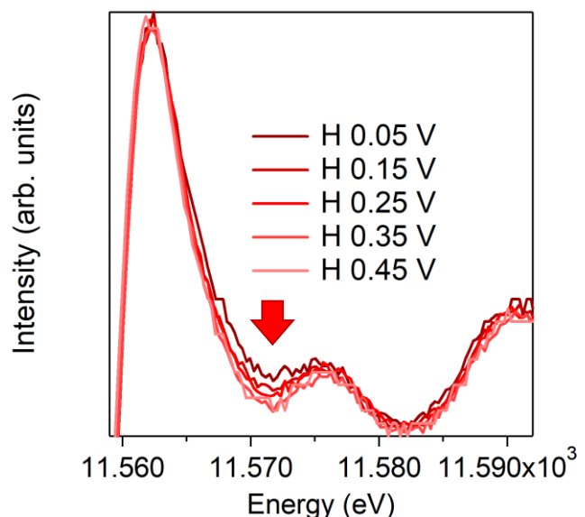
Figure1. Ni 修飾 Pt ナノ粒子の PtLIII edge XANES スペクトル
