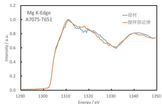
Fig. 2 A7075-T651 の XANES スペクトル
