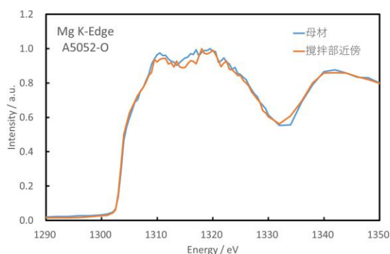
Fig. 1 A5052-O の XANES スペクトル
