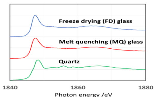
Fig.1 FD 法と MQ 法により作成したホウケイ酸ナトリウムガラスの XANES スペクトル
