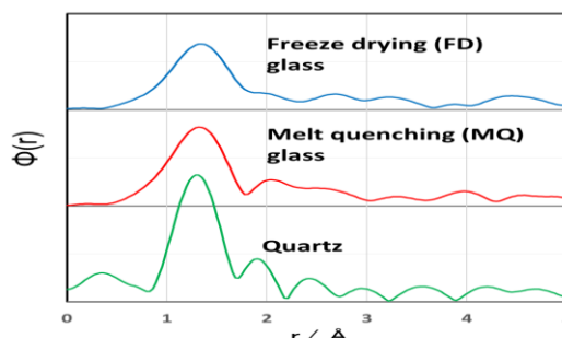
Fig.2 FD 法と MQ 法により作成したホウケイ酸ナトリウムガラスの動径構造関数
